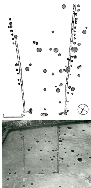
Půdorys domu z mladšího neolitu, podle kterého byla zhotovena rekonstrukce. Podle Pleinerová 1984.
