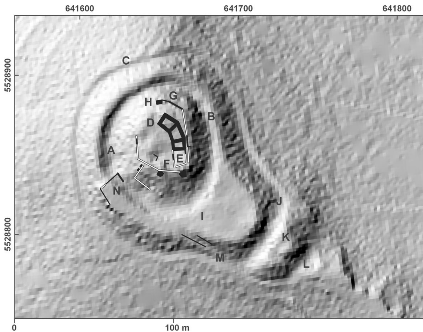
Plán lokality a LLS snímek.
