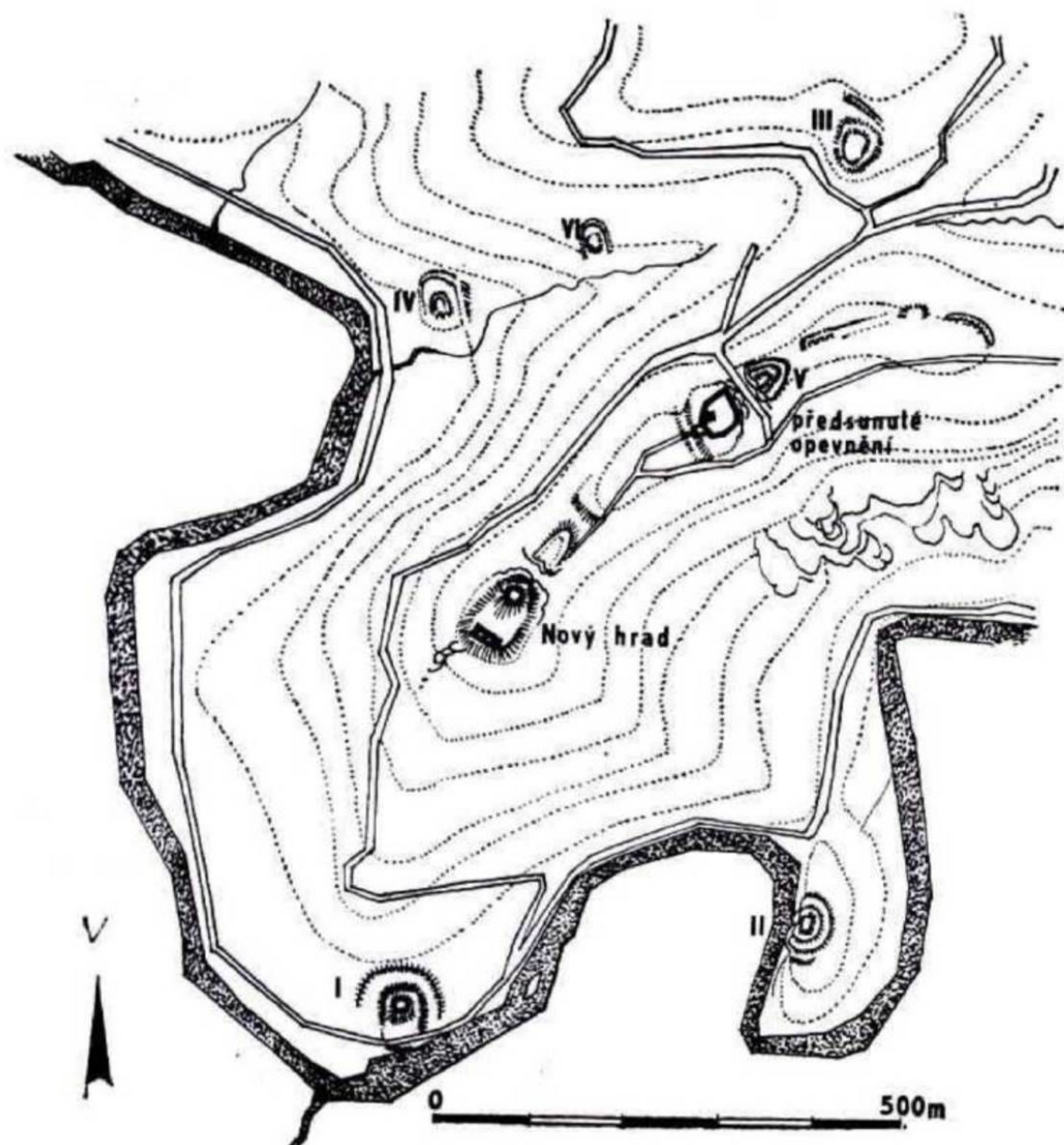
Plán obou hradů a polních opevnění.
