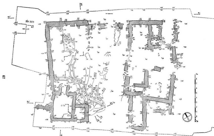
62a. Pfaffenschlag. Půdorys domů IX a X
