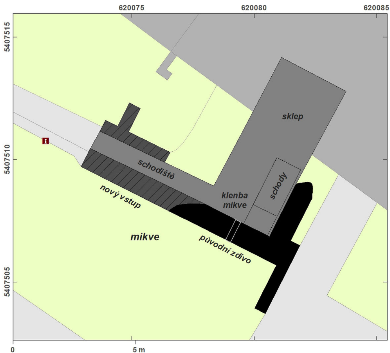
Site plan.
